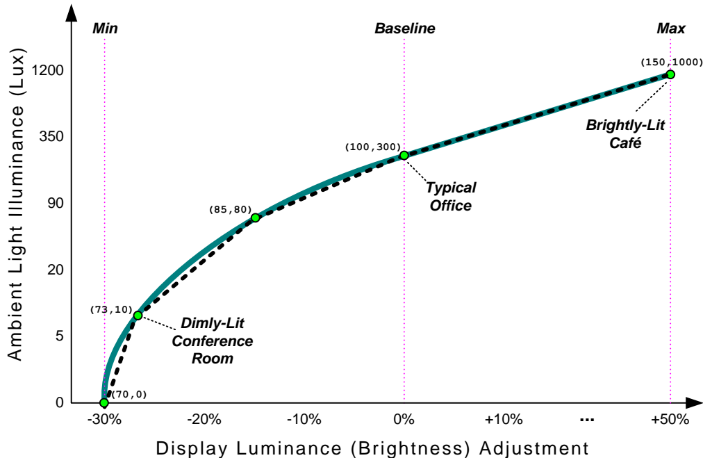
Figure 9-1: A five-point ALS Response Curve
