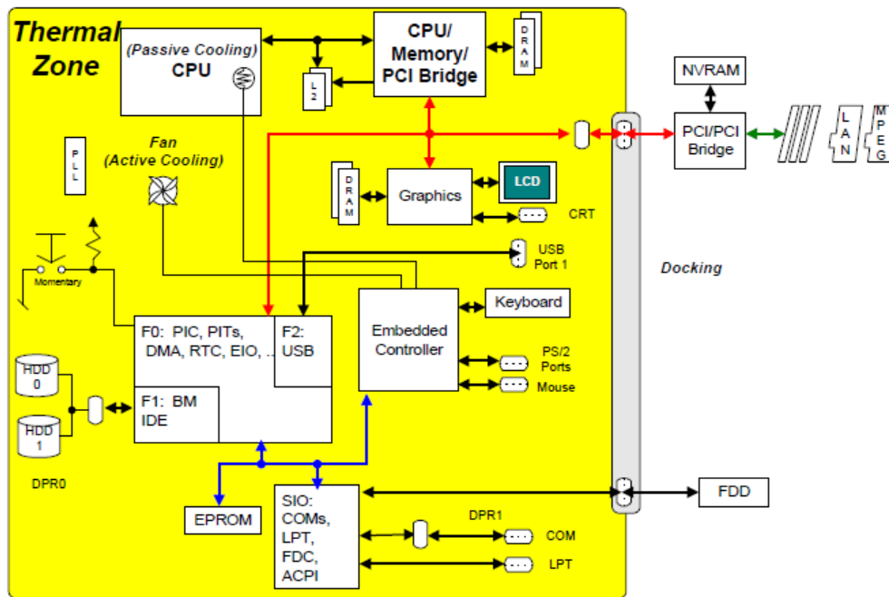
Fig. 3.7: Thermal Zone
