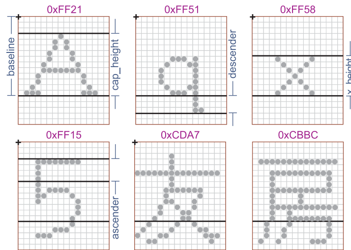
Figure 112. 16 x 19 Font Parameters
