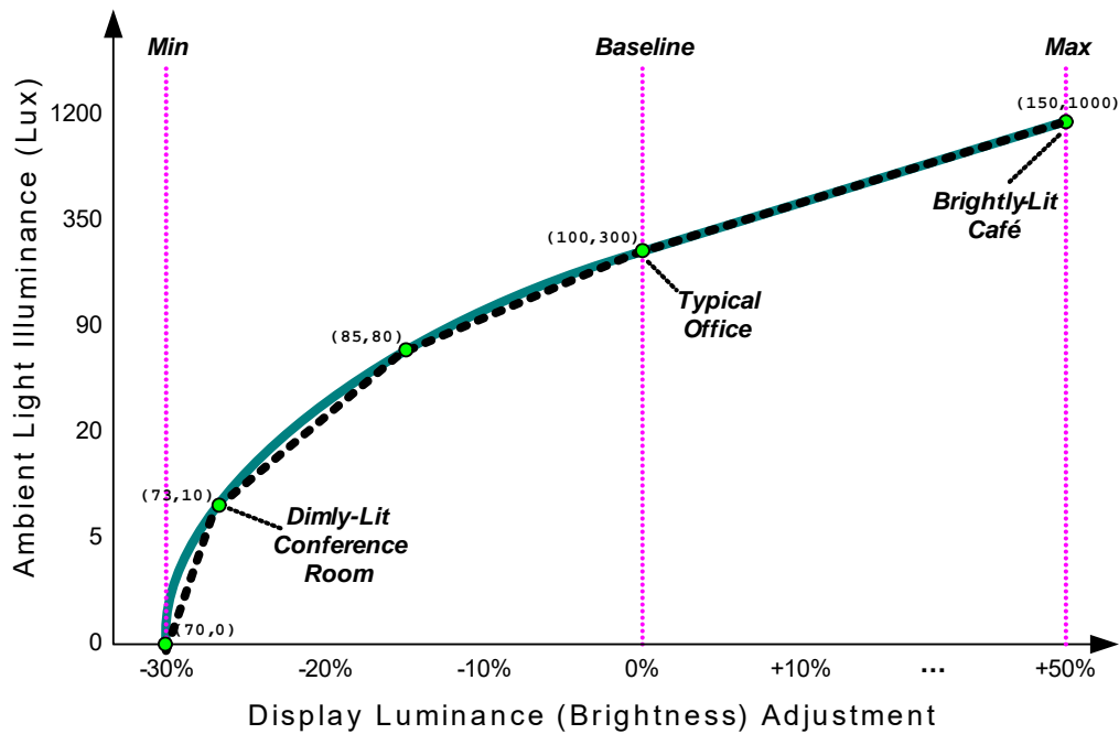
Figure 9-52 A five-point ALS Response Curve
